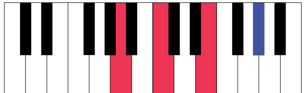
Am maj7
