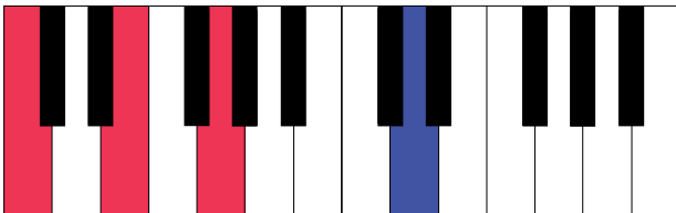
Cadd9
